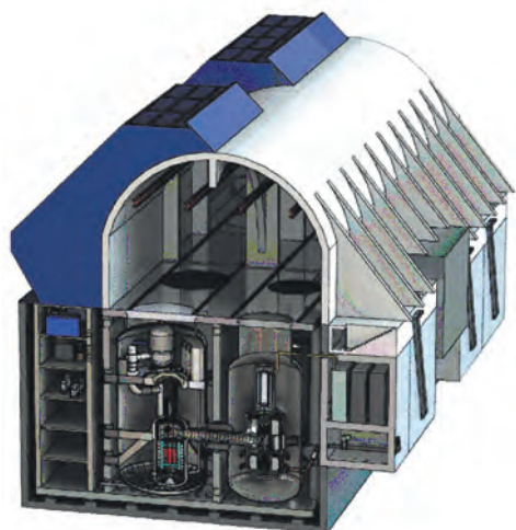
Концепция АЭС с двумя реакторами EM 2
