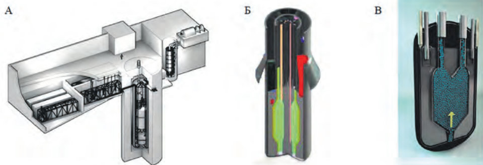
Модели АЭС с реактором типа LFTR (А), а также установок Mk1 PB-FHR (Б) и KP-FHR (В)
