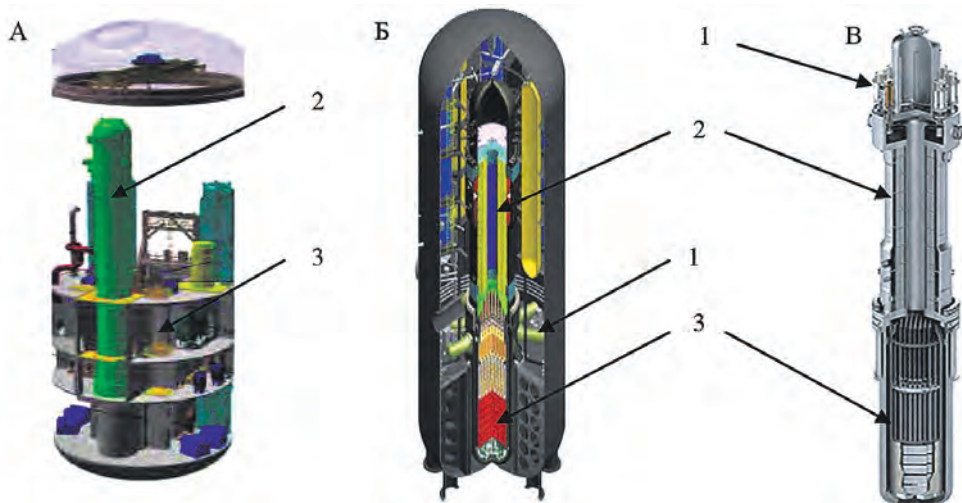
Модели реакторов SMR-160 (А), W-SMR (Б) и mPower (В): 1 – циркуляционные насосы; 2 – парогенератор; 3 – активная зона
