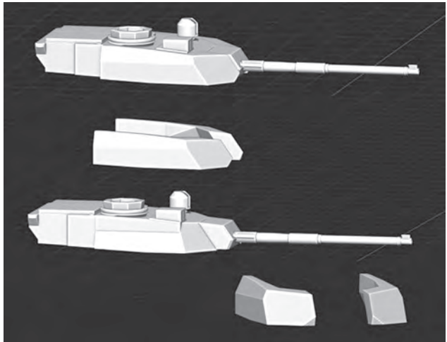
Варианты башенных систем для легкого танка с автоматом заряжания в нише башни
