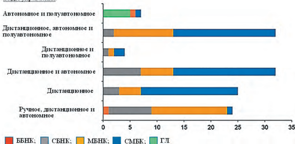
Виды управления существующих ББНК (в ед.)
