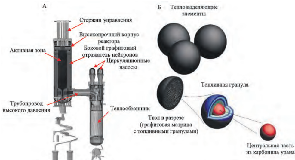
Модель реактора Xe-100 (А) и топлива для него (Б)
